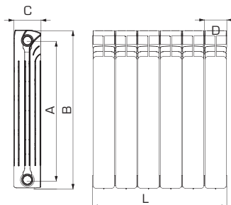
Рис. 1. Габаритные размеры радиатора
